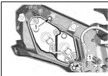
1. Justeringskruen
