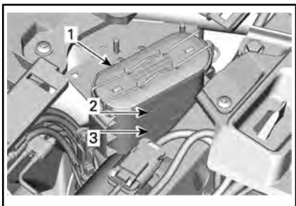
1. Bremsevæskebeholder 2. MAX 3. MIN
