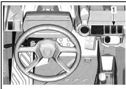
1. Differensiallås bryter
