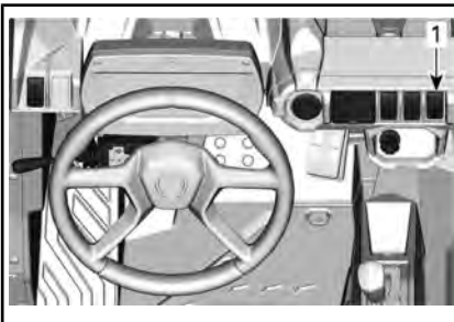
1. Commutateur HDC
