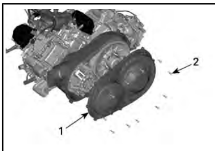
1. Couvercle de la boîte de vitesses CVT 2. Vis du couvercle de la boîte de vitesses CVT
