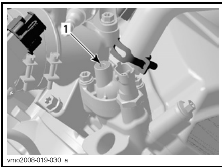
1. Termostathusöppning
