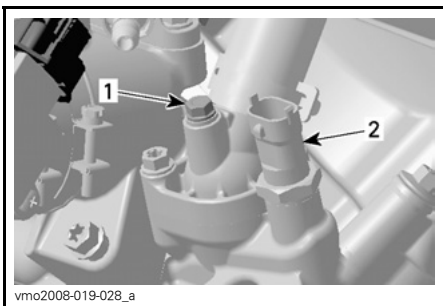
1. Luftningskruv 2. Motortemperaturgivare
