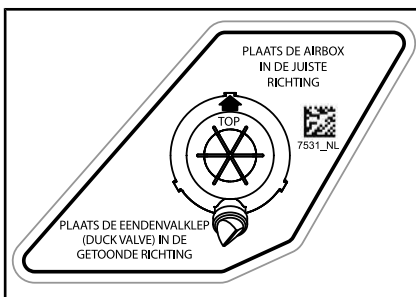
LOCATIE: OP DEKSEL MOTORLUCHTFILTERHUIS
