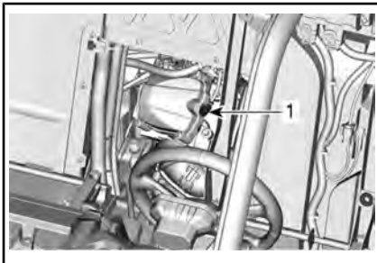
1. Voorste bougie
