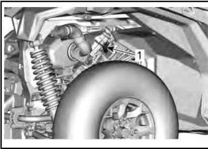
1. Ontstekingsbougie
