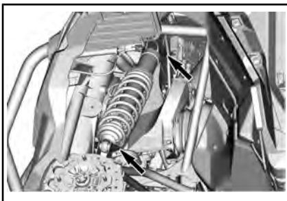
ONDERDELEN VERWIJDERD VOOR DE OVERZICHTELIJKHEID - VOORSTE SCHOKDEMPERBEVESTIGINGEN
