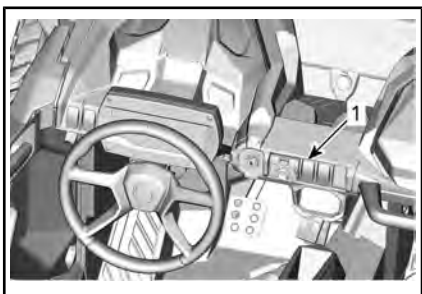
1. Schakelaar 2WD/4WD/Voordifferentieelvergrendelaar
