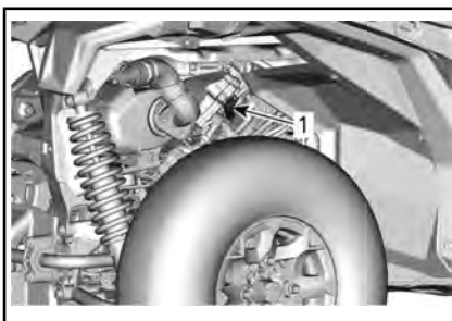
1. Bougie arrière
