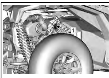
1. Bougie
