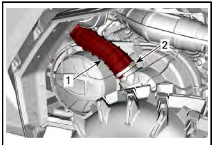
1. Tubo di aspirazione aria CVT.
