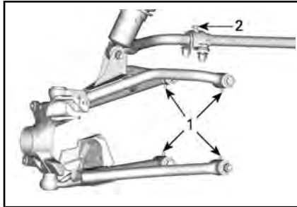
SUSPENSIÓN DELANTERA
