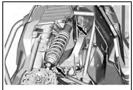
ONDERDELEN VERWIJDERD VOOR DE OVERZICHTELIJKHEID - VOORSTE SCHOKDEMPERBEVESTIGINGEN
