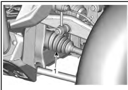
1. Manchetten binnenkant aandrijfjas
