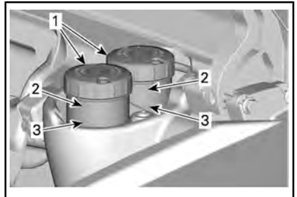
1. Serbatoi del liquido per freni 2. MAX 3. MIN
