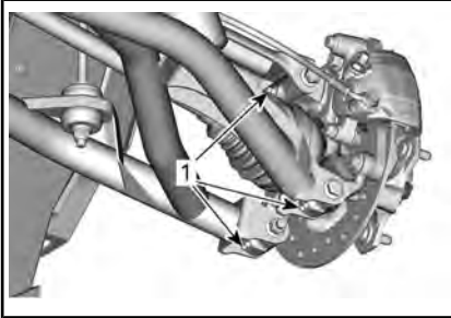
1. Punti di ingrassaggio degli snodi posteriori
