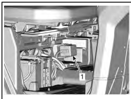
COPERCHIO DELLA BATTERIA RIMOSSO
