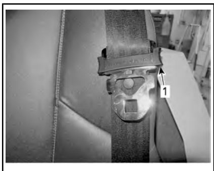
1. Linguetta di pretensionamento
