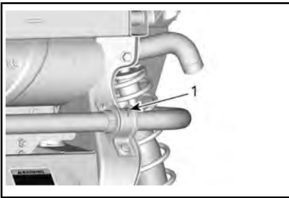
1. Punto di ingrassaggio della boccola della barra stabilizzatrice posteriore
