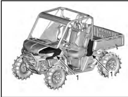
1. Sujeciones inferiores de la jaula
