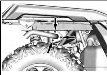
TORNILLOS DE SUJECIÓN DEL TUBO DE ESCAPE
