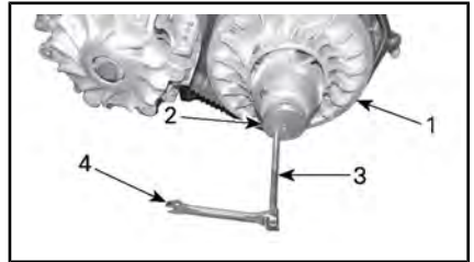
SEQUÊNCIA DE APERTO DA TAMPA DA CVT
