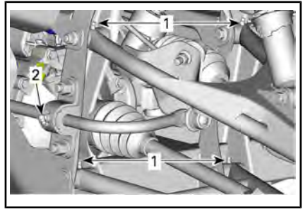
SUSPENSÃO DIANTEIRA - TÍPICA
