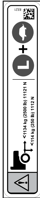
ÉTIQUETTE 11 - HD8 ET HD10
