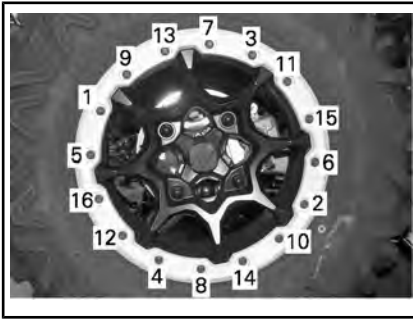
ТИПОВОЙ ВАРИАНТ - ПОРЯДОК ЗАТЯЖКИ ВИНТОВ
