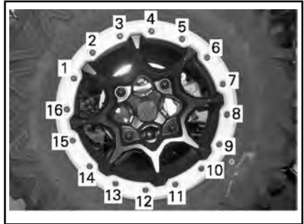
ТИПОВОЙ ВАРИАНТ - ЗАКЛЮЧИТЕЛЬНЫЙ ЭТАП ЗАТЯЖКИ ВИНТОВ
