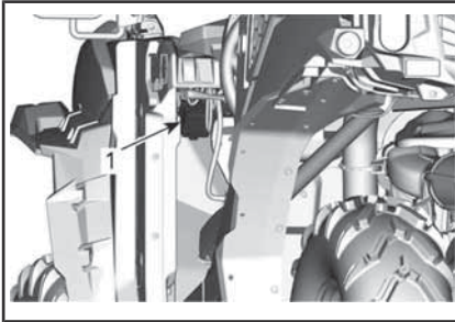
1. Scatola fusibili anteriore
