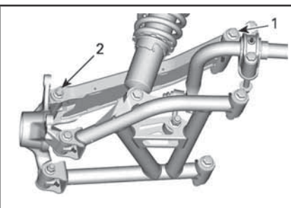
1. Dado flangiato elastico M12
