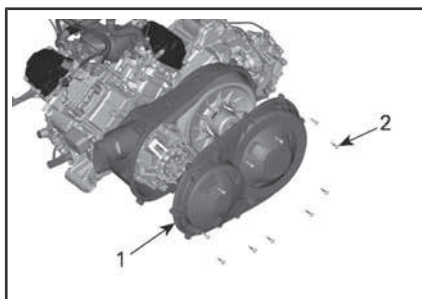
1. Carenatura CVT 2. Viti della carenatura CVT
