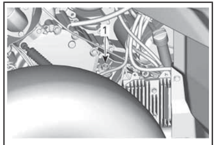
1. Växellådans oljenivåplugg
