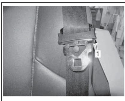
1. Låsspärr
