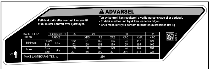
DEKAL 5
