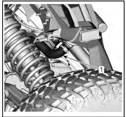
1. Nedre slange
