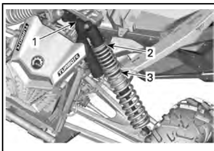
TYPISK – MAVERICK TURBO OG X rc TURBOMODELLER – FJÆRING FORAN
