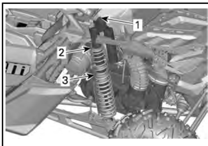
TYPISK – MAVERICK TURBO OG X rc TURBOMODELLER – FJÆRING BAK
