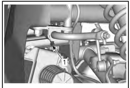
SITUAZIONE TIPICA - BARRA STABILIZZATRICE ANTERIORE
