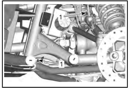
SITUAZIONE TIPICA - SOSPENSIONE ANTERIORE
