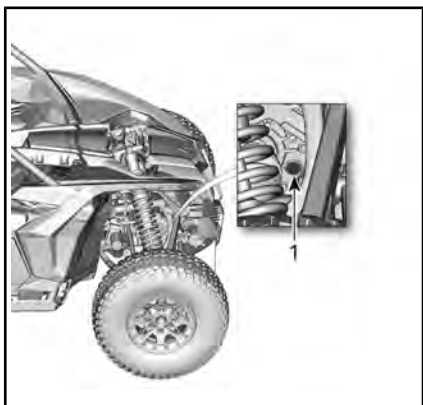
1. Tappo livello olio scatola del cambio.
