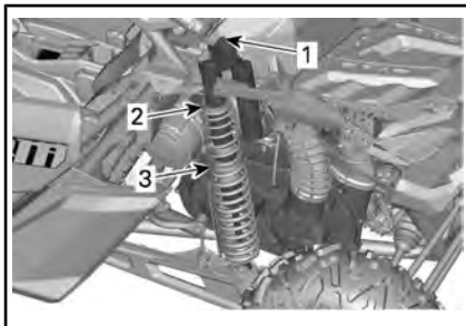
CONFIGURAZIONE TIPICA - MODELLI MAVERICK TURBO E X rc TURBO - SO-SPENSIONE POSTERIORE
