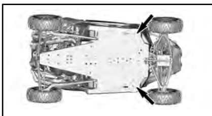
POSIZIONI DEL MARTINETTO - LATO ANTERIORE DEL VEICOLO
