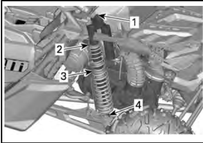
CONFIGURAZIONE TIPICA - MODELLI MAVERICK MAX X ds - SOSPENSIONE POSTERIORE
