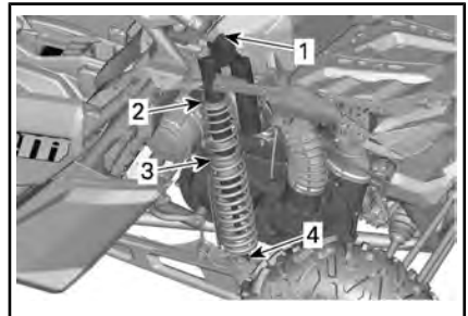
典型示例 - Maverick x ds 型号 - 后悬架
