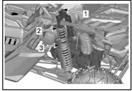
典型示例 - Maverick Turbo 和 X rc Turbo 型号 - 后悬架
