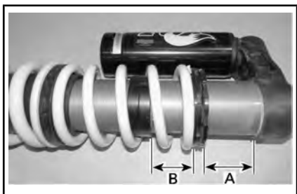
典型示例 - 交叉调整 - 后减震器
