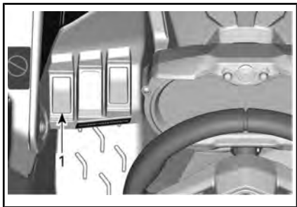
1. 绞盘开关
