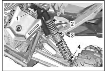
典型示例 - MAVERICK X ds、X rs 和 XRC TURBO r 型号 - 前悬架
