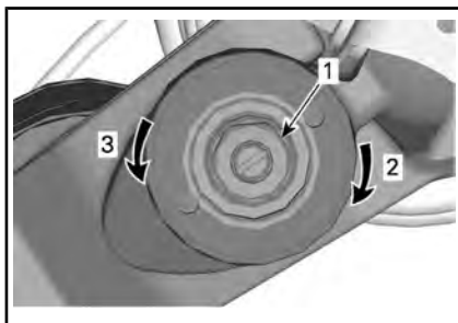
高速压缩阻尼 (使用 17 mm 螺丝刀)
