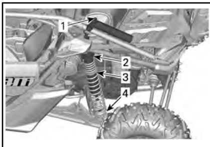
ESEMPIO TIPO: MODELLI MAVERICK MAX X RS - SOSPENSIONE POSTERIORE
