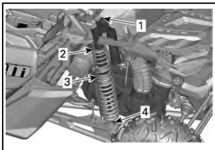
ESEMPIO TIPO: MODELLI MAVERICK MAX X DS - SOSPENSIONE POSTERIORE
