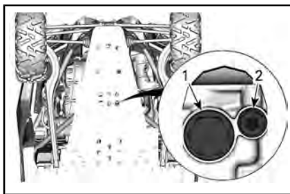
SOTTO LA PARTE POSTERIORE DEL VEICOLO
