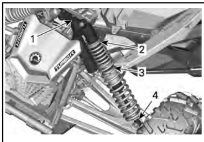
ESEMPIO TIPO: MODELLI MAVERICK MAX X DS E X RS - SOSPENSIONE ANTERIORE
