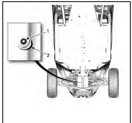
MODELLI CON DIFFERENZIALE ANTERIORE SMART-LOK
