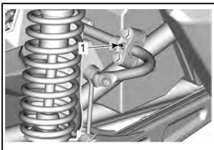
SITUAZIONE TIPICA - BARRA STABILIZZATRICE POSTERIORE
