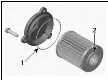
COPERCHIO DI MANUTENZIONE ANTERIORE
