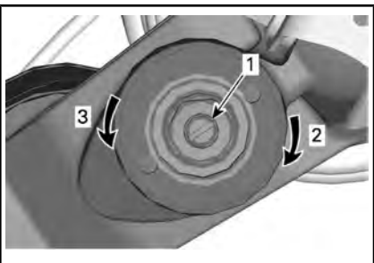
低速压缩阻尼 (使用螺丝刀)
