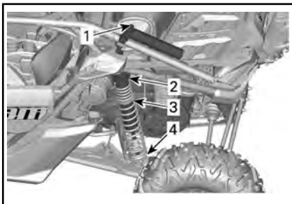
典型示例 - Maverick MAX X rsrs 车型 - 后悬架
