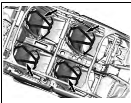
典型示例 - 为方便观察已拆下部分零件
