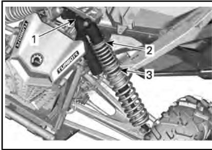
典型示例 - Maverick MAX 车型 - 前悬架
