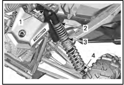
典型示例 - Maverick MAX x dsds 和 x rsrs 车型 - 前悬架
