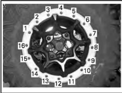
典型示例 - 最终紧固顺序
