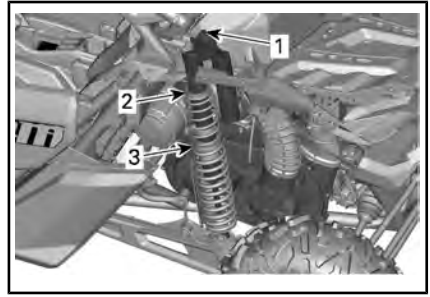
典型示例 - Maverick MAX 车型 - 后悬架
