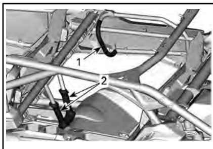
后扶手
