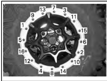
典型示例 - 紧固顺序
