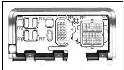
ZEKERINGSDOOSBEVESTIGING
