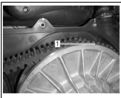
1. Het onderste deel van de tangen gelijk met de buitenkant van de aandrijfriem
