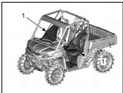
1. Zijnet
