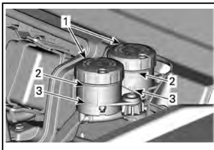
1. Reservatórios de fluido de freio 2. MÁX. 3. MÍN.
