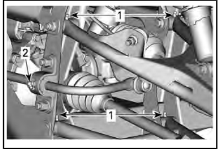
SUSPENSÃO DIANTEIRA - TÍPICA
