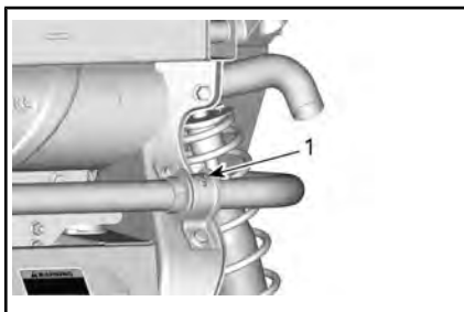
1. Graxeira da bucha da barra estabilizadora traseira
