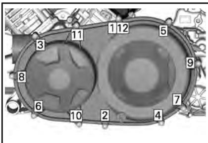
AANDRAAIVOLGORDE CVT-DEKSEL HD8
