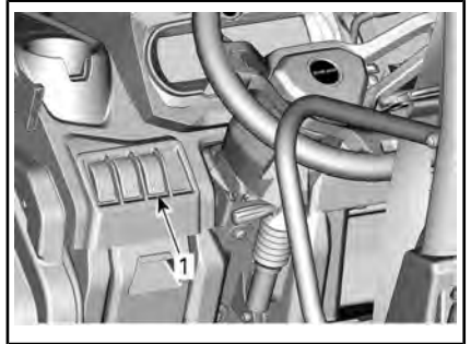
1. Claxonschakelaar
