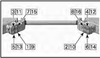
SECUENCIA DE APRIETE DE LA BARRA ESTABILIZADORA
