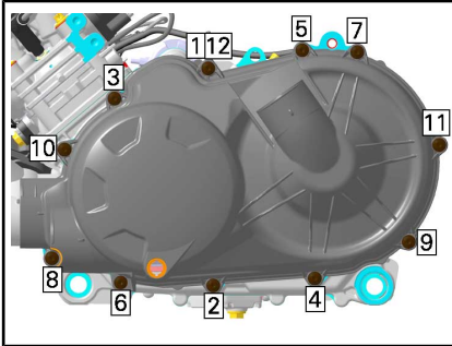
HD5 - STRAMMEREKKEFØLGE FOR CVT-DEKSEL
