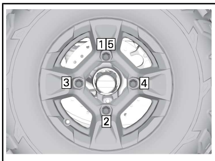
TILTREKKINGSREKKEFØLGE
