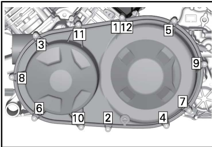
HD8 OG HD10 - STRAMMEREKKEFØLGE FOR CVT-DEKSEL
