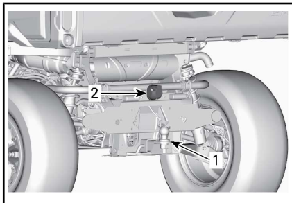
1. Tilhengerfeste 2. Tilhengerkontakt
