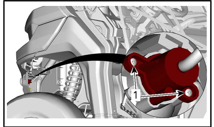
SOKKEL FOR BLINKLYS
