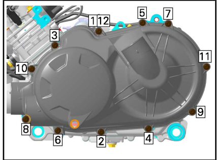
HD5 – CVT:N (PORTAATON VOIMANSIIRTO) KANNEN KIRISTÄMISJÄRJESTYS
