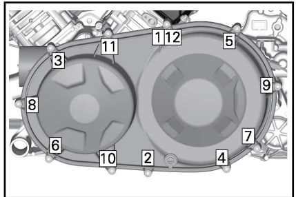
HD8 JA HD10 – CVT:N (PORTAATON VOIMANSIIRTO) KANNEN KIRISTÄMISJÄRJESTYS
