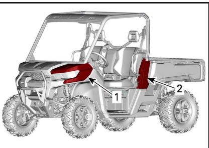
1. Kehikon alakiinnittimet
