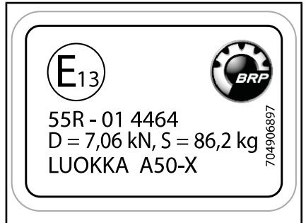
VETOKOUKUSSA
