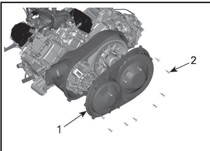
1. Carenatura CVT 2. Viti della carenatura CVT
