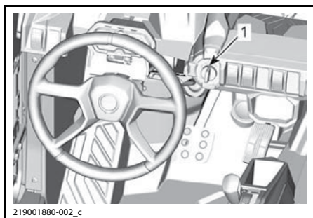
1. Замок зажигания
