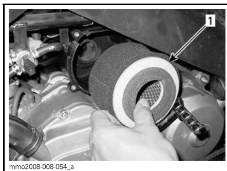
DEMONTERA LUFTILTRET FRÅN KÅPAN 1. Luftfilter
