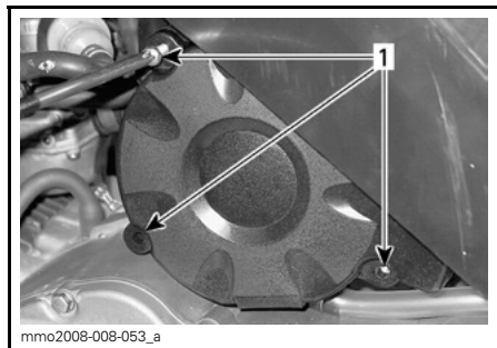
DEMONTERA LUFTFILTERKÅPAN 1. Skruvar
