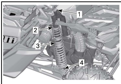
TYPISCH - MAVERICK X dsDS-MODELLEN - OPHANGING ACHTER
