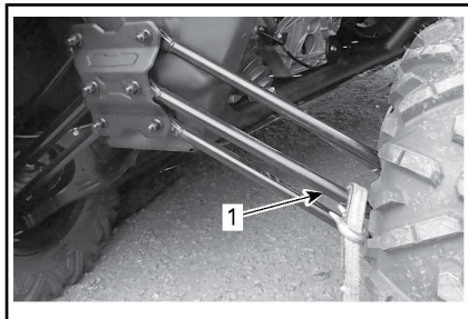
1. Ophangingsarm middenachter
