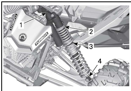
TYPISCH - MAVERICK X dsDS, XrsRS EN XRCRC TURBO R MODELLEN - OPHANGING VOOR
