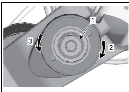
COMPRESSIEDEMPING BIJ HOGE SNELHEID (GEBUIK EEN SLEUTEL VAN 17 MM)
