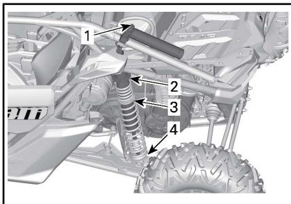
TYPISCH - MAVERICK XrsRS EN XRCRC TURBO R MODELLEN - OPHANGING ACHTER
