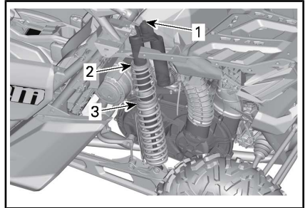
TYPISCH - MAVERICK TURBO EN X RC TURBO MODELLEN - OPHANGING ACHTER
