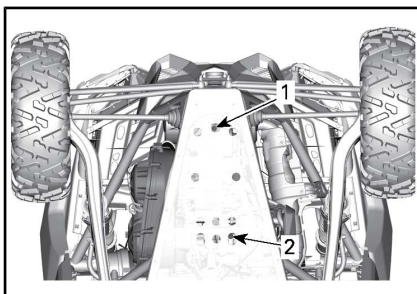
1. Aftapplug tandwielkast 2. Motorolieaftapplug
