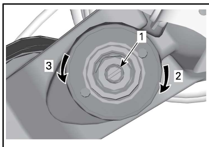
COMPRESSIEDEMPING BIJ LAGE SNELHEID (GEBUIK EEN SCHROEVENDRAAI-ER)
