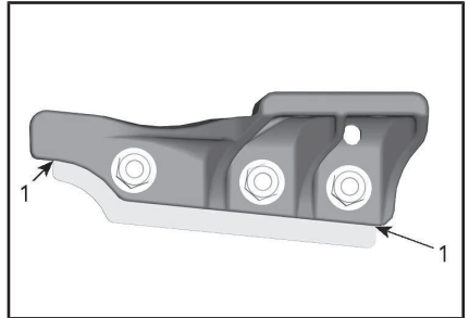
1. 磨损极限
