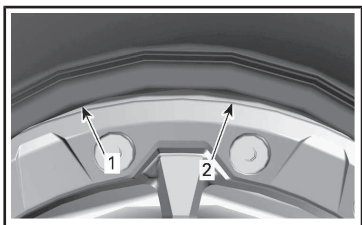
典型示例 轮胎外胎圈 防脱圈内环凸肩
