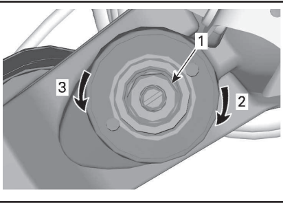
高速压缩阻尼（使用 17 mm 螺丝刀）
