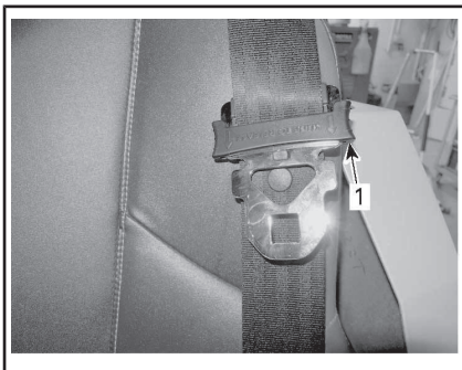
1. 滑动锁定片
