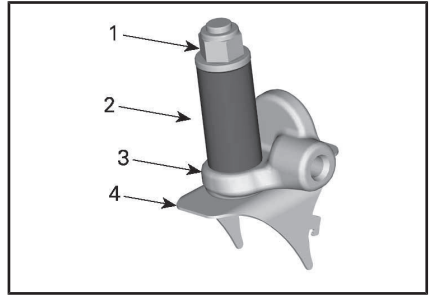
高位后锚点
