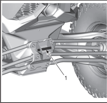
1. 后部挂接钩
