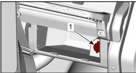
МОДЕЛИ С СИСТЕМОЙ ОБОГРЕВА 1. Электрические розетки (12 В)
