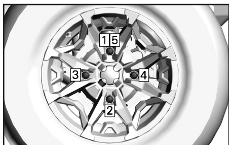
ПОСЛЕДОВАТЕЛЬНОСТЬ ЗАТЯЖКИ
