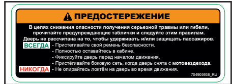
НАКЛЕЙКА 20 — МОДЕЛИ С КАБИНОЙ
