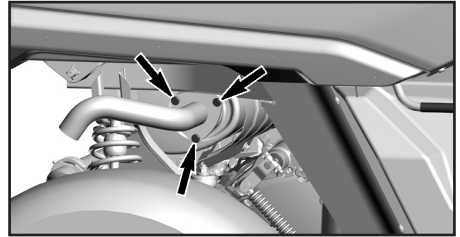
ВИНТЫ И ГАЙКИ КРЕПЛЕНИЯ ВЫХЛОПНОЙ ТРУБЫ
