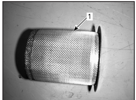
1. Очистите искрогаситель
