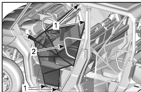
1. Расположение регулировочных элементов боковой сети 2. Защита плечевого пояса
