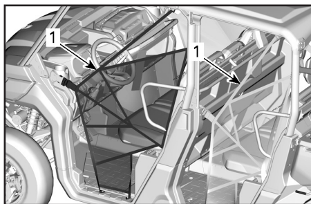
1. Боковая сеть
