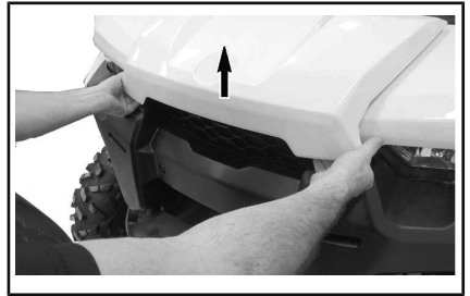
SOULEVER LA BORDURE DU COUVERCLE D'ENTRETIEN AVANT.
