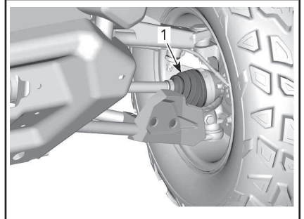
1. Soufflets d'arbre de transmission intérieur
