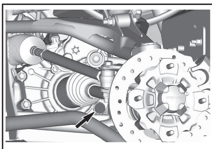
TYPIQUE SMART-LOC -- CÔTÉ DROIT AVANT DU VÉHICULE
