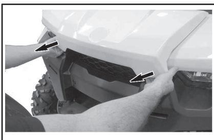
TIREZ SUR LA BORDURE DU COUVERCLE D'ENTRETIEN AVANT.
