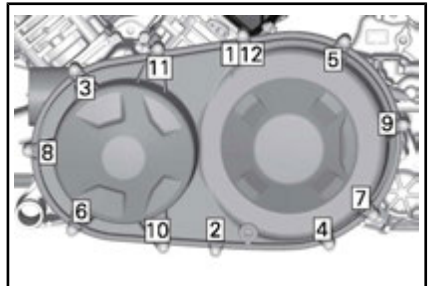
AANDRAAIVOLGORDE CVT-DEKSEL
