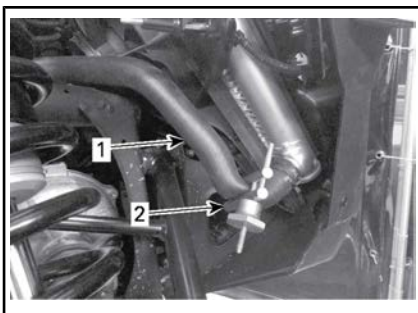
1. Unterer Schlauch des Kühlers 2. Schlauchklemme
