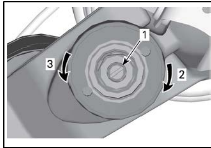
EINFEDERUNGSDÄMPFUNG (NIEDRIGE GESCHWINDIGKEIT), (EINEN SCHRAUBENDREHER VERWENDEN)
