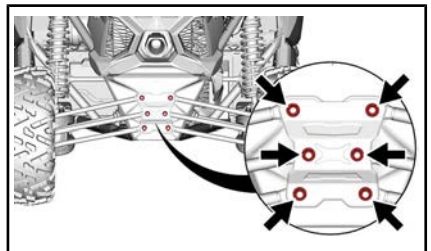
TYPISCH — STABILISATORSTANGE VONR
