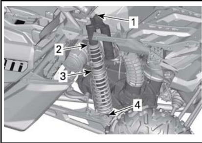
TYPISCH - MAVERICK X3 MAX X dsDS MODELLE - HINTERRADAUFHÄNGUNG
