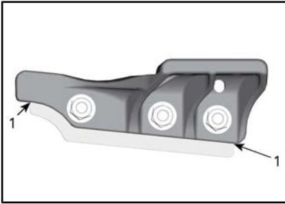
1. Verschleißgrenze
