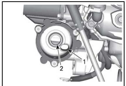
1. Auslass zur Ölspeisung des Motors 2. Einlass der Ölpumpe zum Ölfilter
