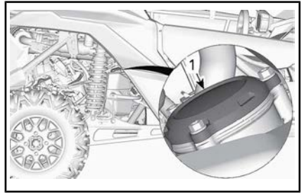
1. Ölfilterdeckel
