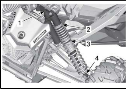
TYPISCH - MAVERICK X3 MAX X dsDS UND X rsRS MODELLE - VORDERRADAUFHÄNGUNG
