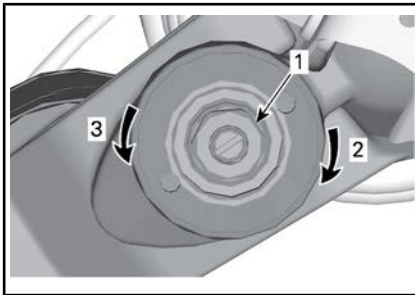
EINFEDERUNGSDÄMPFUNG (HOHE GESCHWINDIGKEIT), (EINEN 17-MM-SCHRAUBENSCHLÜSSEL VERWENDEN)
