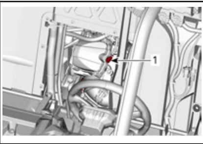
1. Vela de ignição dianteira
