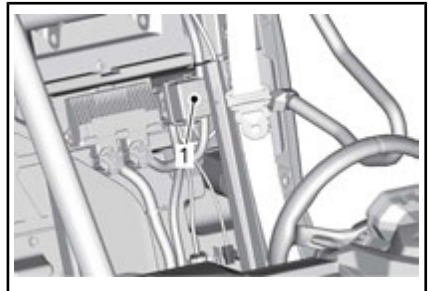
1. Zekeringdoos achter
