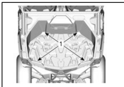
1. Ankerhaken
