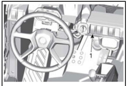
1. Keuzeschakelaar 2WD/4WD
