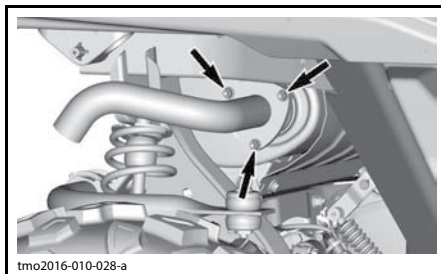
ТИПОВОЙ ВАРИАНТ — ВИНТЫ И ГАЙКИ КРЕПЛЕНИЯ ВЫХЛОПНОЙ ТРУБЫ
