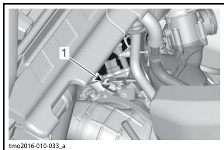
ПЕРЕДНИЙ ЦИЛИНДР (ЛЕВАЯ СТОРОНА) 1. Свеча зажигания
