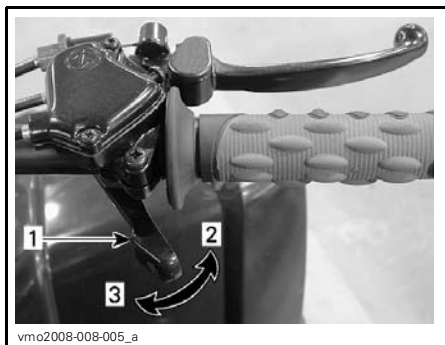
1. Levier d'étrangleur 2. Pour accélérer 3. Pour décélérer
