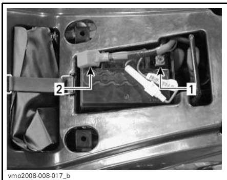
1. Porte-fusible
