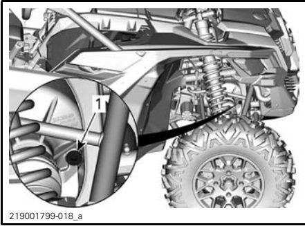
1. Filler plug
