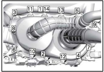
Típico - SEQUÊNCIA DE APERTO DA TAMPA DA CVT
