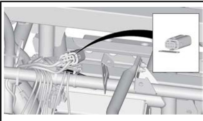
TERCEIRA CAIXA DE FUSÍVEIS - ATRÁS DO CONSOLE SUPERIOR
