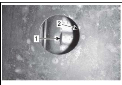
1. Bujão de drenagem do óleo 2. Abertura na placa de proteção do cárter
