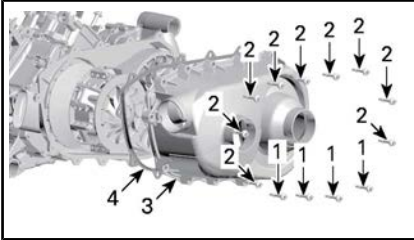
Típico - SEQUÊNCIA DE APERTO DA TAMPA DA CVT
