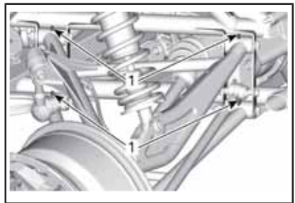
HINTERE AUFHÄNGUNG - TYPISCH
