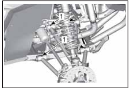
VORDERRADAUFHÄNGUNG - TYPISCH
