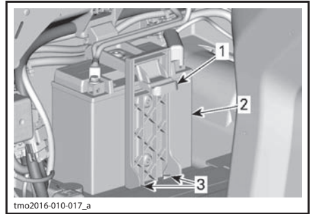
1. Держатель аккумуляторной батареи 2. Аккумуляторная батарея 3. Винты крепления держателя аккумуляторной батареи
