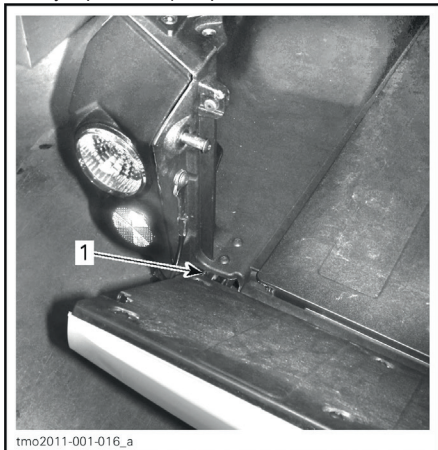
1. Петля верхнего откидного борта
