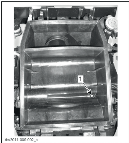
1. Сливное отверстие
