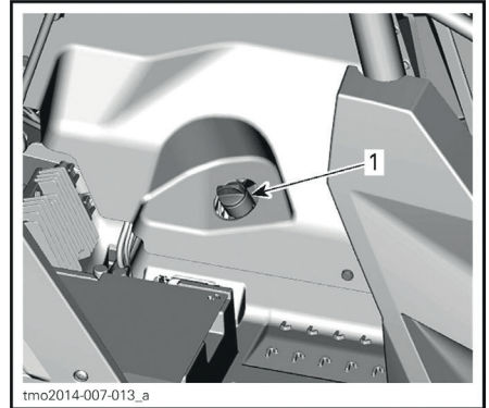
НЕКОТОРЫЕ ДЕТАЛИ СНЯТЫ ДЛЯ НАГЛЯДНОСТИ 1. Щуп
