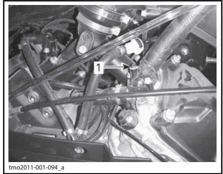
ТИПОВОЙ ВАРИАНТ 1. Сливной винт
