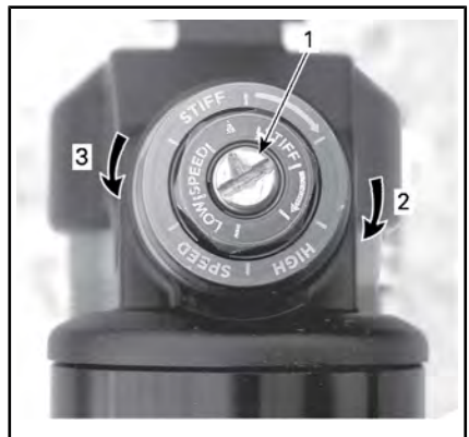
AMORTIGUACIÓN DE COMPRESIÓN A VELOCIDAD BAJA (UTILICE UN DESTORNILLADOR)
