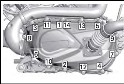
SECUENCIA DE APRIETE DE LA TAPA DE LA CVT - ASPIRACIÓN NATURAL
