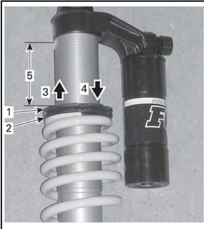
TÍPICO - SE MUESTRA EL AMORTIGUADOR DELANTERO
