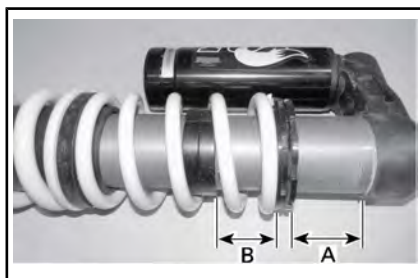
AMORTIGUACIÓN DE COMPRESIÓN A VELOCIDAD ALTA (UTILICE UNA LLAVE DE 17 MM)
