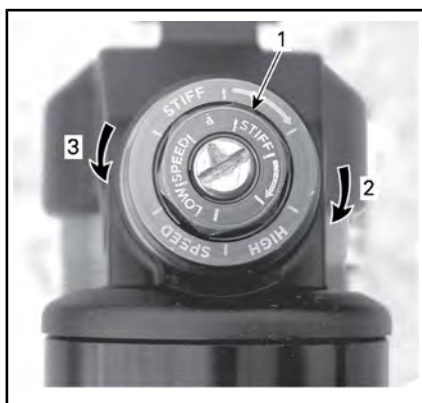
AMORTIGUACIÓN DE COMPRESIÓN A VELOCIDAD ALTA (UTILICE UNA LLAVE DE 17 MM)
