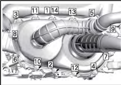
SECUENCIA DE APRIETE DE LA TAPA DE LA CVT - MODELO TURBO
