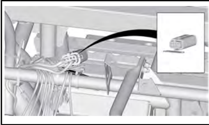
TERCERA CAJA DE FUSIBLES, TRAS LA CONSOLA SUPERIOR, EN MODELOS TURBO
