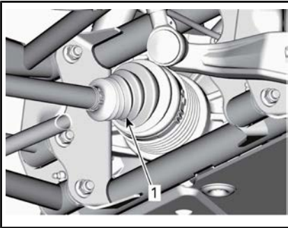
VANLIG – KJØRETØYETS BAKSIDE (KOMponenter fjernet for bedre innsikt)
