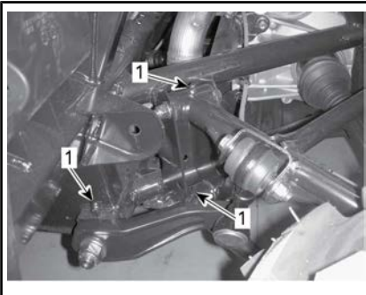
FJÆRING BAK – TYPEBILDE
