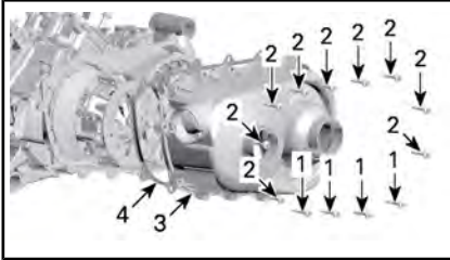
AANDRAAIVOLGORDE CVT-DEKSEL
