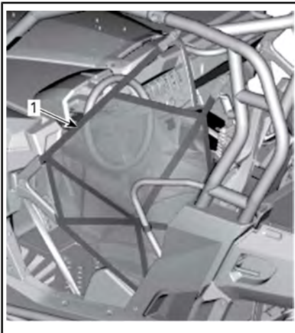
1. Zijnet
