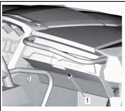
1. Vergrendeling handschoenvak
