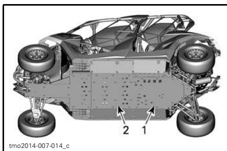
1. Plaque de protection arrière 2. Plaque de protection centrale
