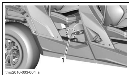
tmo2016-003-004_a TYPIQUE - EMPLACEMENT DES FILS FUSIBLES ET DE LA BOÎTE À FUSIBLE 3 SUR LE VÉHICULE
