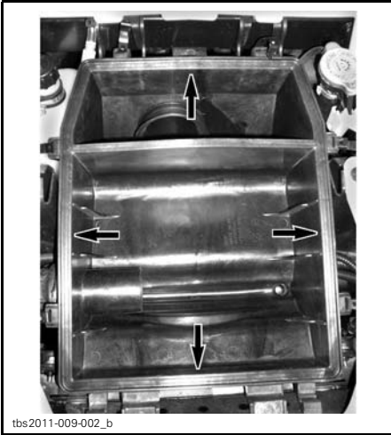
NETTOYEUR DE FILTRE À AIR (N/P 219 700 341)
