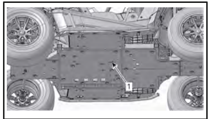
1. Åtkomst till kylsystemets dräneringsplugg
