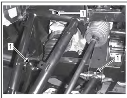
TYPBILD - FRAMFJÄDRING
