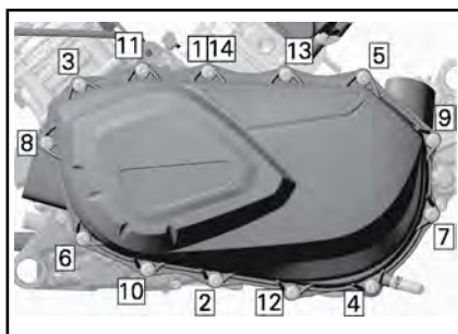
CVT-KÅPANS ÅTDRAGSSEKVENS
